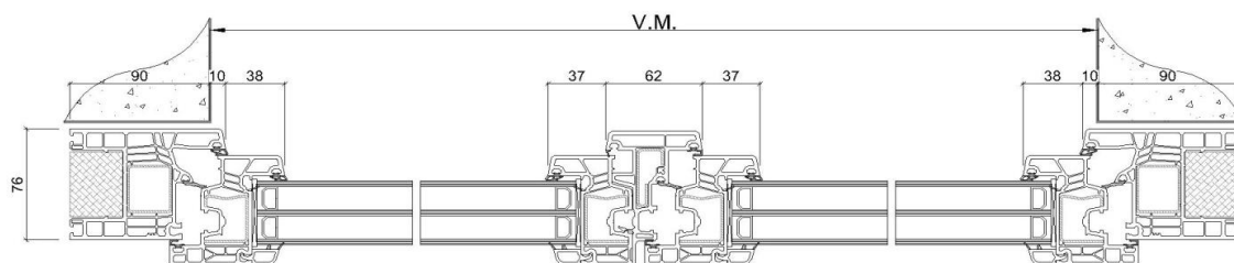
Coupe A-A
