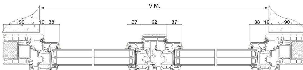
Coupe A-A
