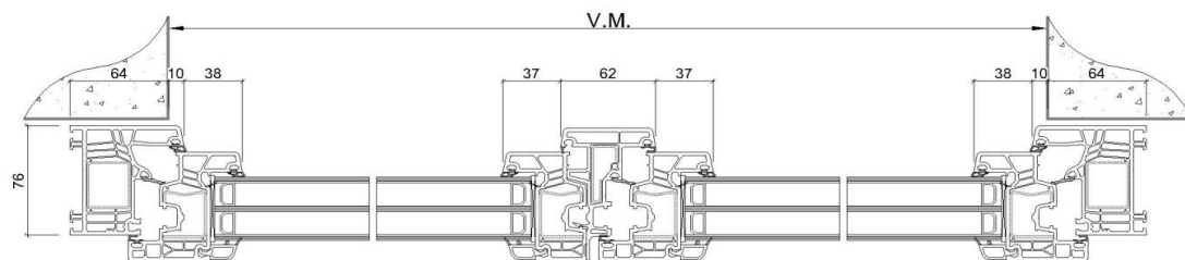
Coupe A-A
