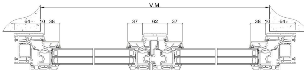
Coupe A-A
