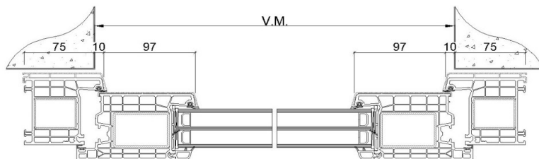
Coupe A-A
