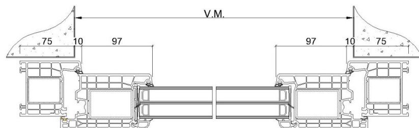
Coupe A-A
